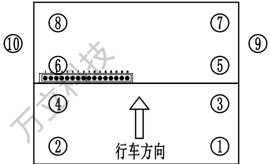
双秤台传感器分布图
